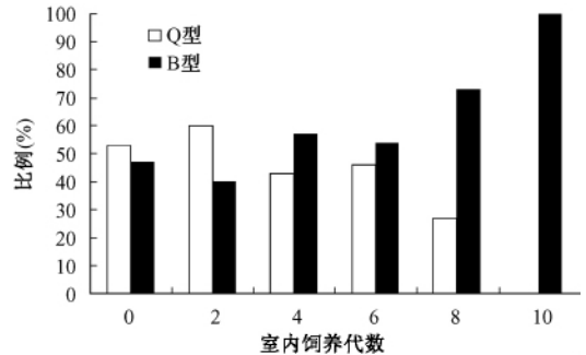
图1 烟粉虱混合种群生物型变化规律
