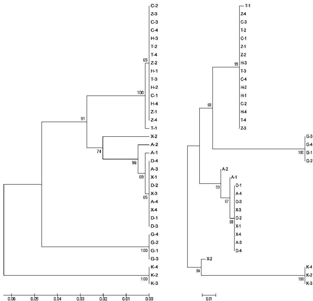
图 2 亚洲小车蝗及外群种 ND1 部分序列 UPGMA 和 NJ 分子系统树
