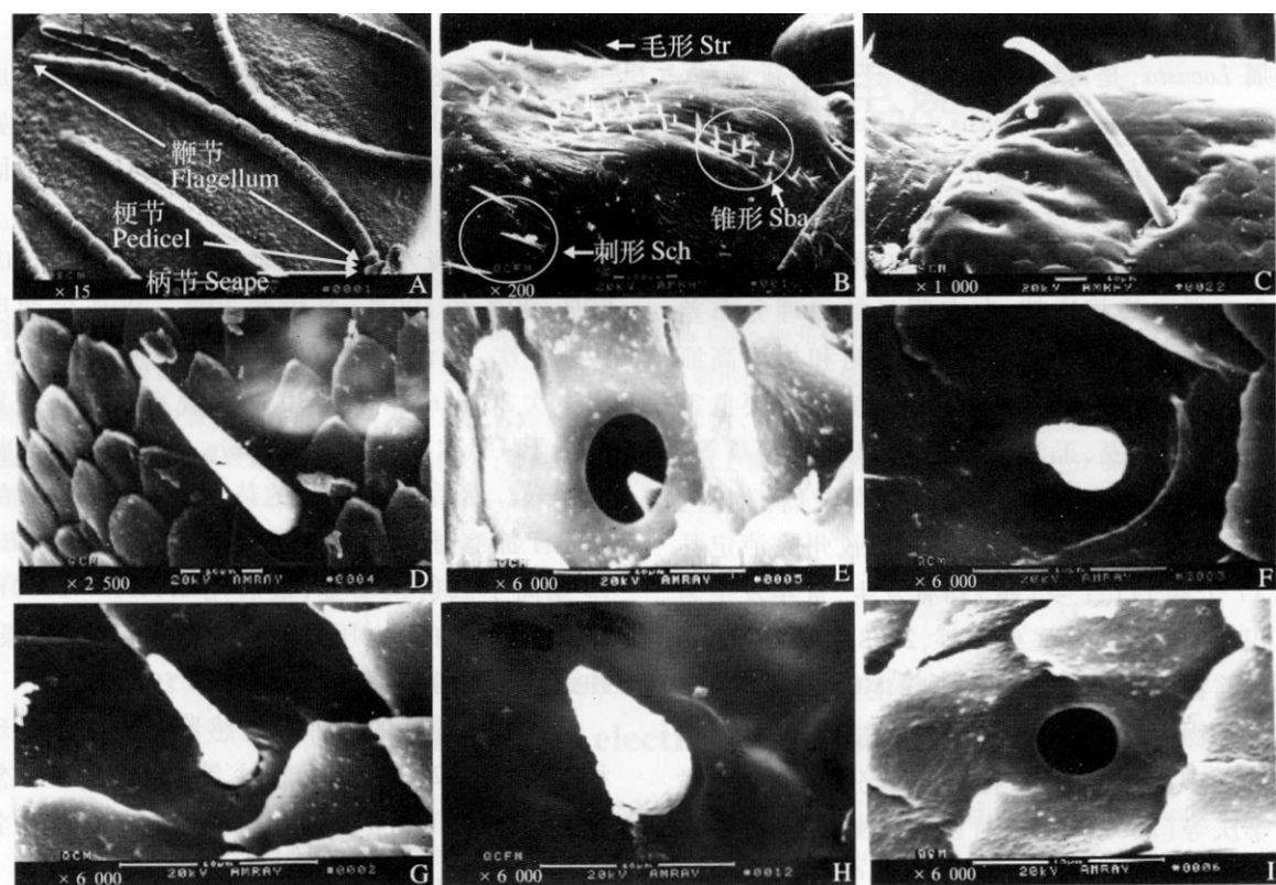
图1 西藏飞蝗触角感器的种类和形态特征
