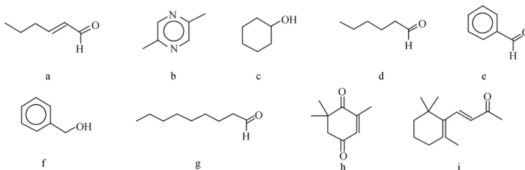
图 3 已报道的东亚飞蝗虫粪挥发物电生理活性组分
