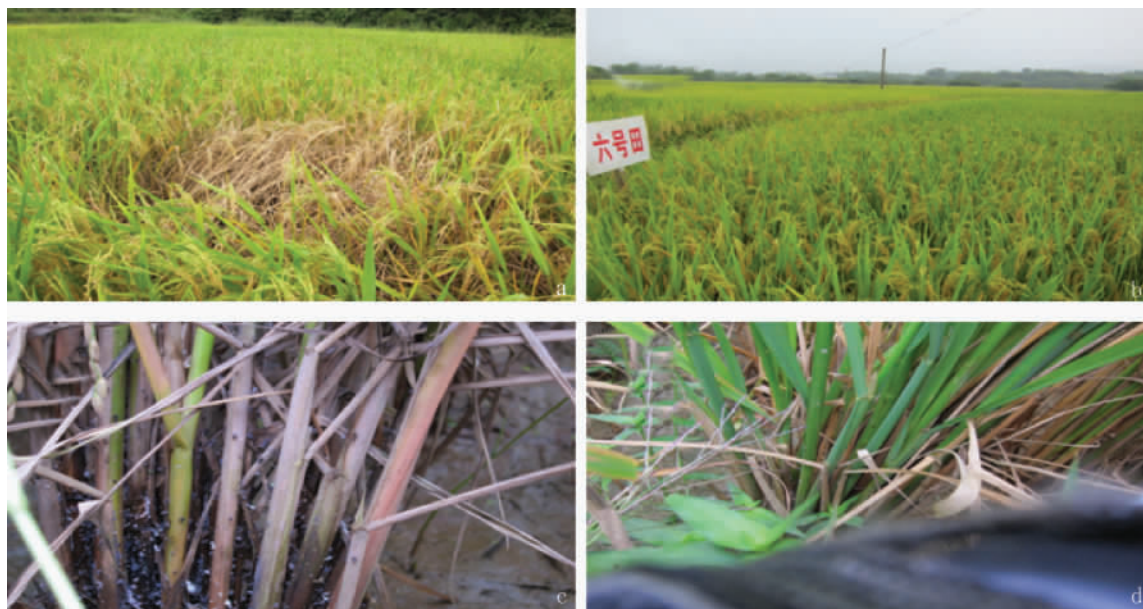
图 3 改良杂交组合川香 29A/华恢 1462 及对照两优培九的田间抗性表现对比
