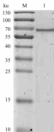
图 4 凝胶过滤层析后取 1 号峰液进行 SDS-PAGE
