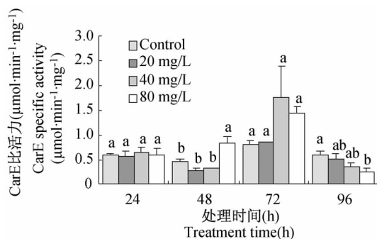
图1 Cd对中华稻蝗 CarE 活性 ( \alpha -NA 为底物) 的影响
