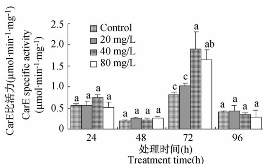
图2 Cd对中华稻蝗 CarE 活性 ( \beta -NA 为底物) 的影响
