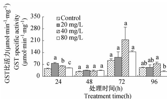
图3 不同 Cd 处理对中华稻蝗 GST 活性的影响
