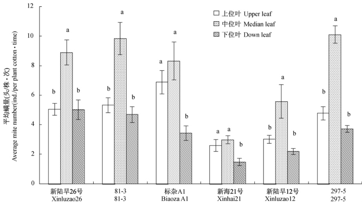
图 2 6 种棉花品种不同叶位土耳其斯坦叶螨数量比较
