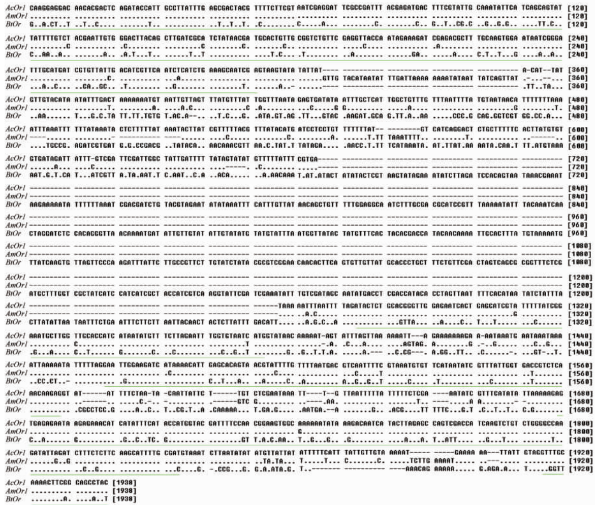
图2 AcOr1 核苷酸序列与其它昆虫相应序列的比对
