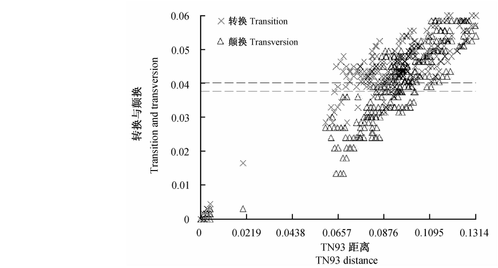
图 2 基于 658 bp 线粒体基因 COI 的序列饱和性分析散点图 Fig.2 Saturation plots for the mitochondrial COI sequences with 658 bp
