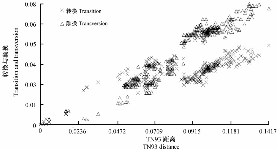
图 1 基于 633 bp 的 COI 序列饱和性分析散点图 Fig.1 Saturation plots for the mitochondrial 633 bp COI sequences
