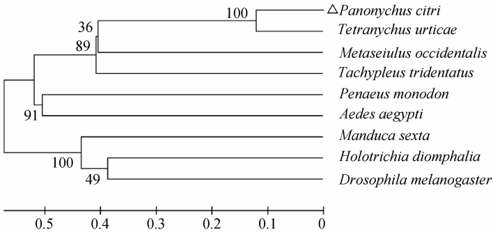
图3 柑橘全爪螨 PPAE 的系统发育树
