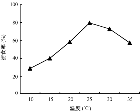
图 2 温度对小十三星瓢虫捕食作用的影响
