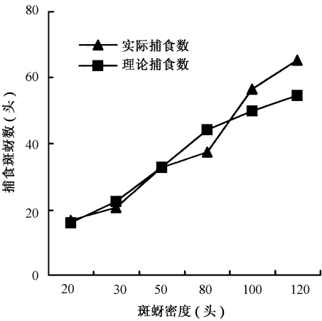
图 1 小十三星瓢虫对不同密度苜蓿斑蚜捕食作用
