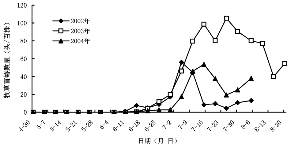
图 1 南疆棉田牧草盲蝽种群季节消长(2002~2004 年)
