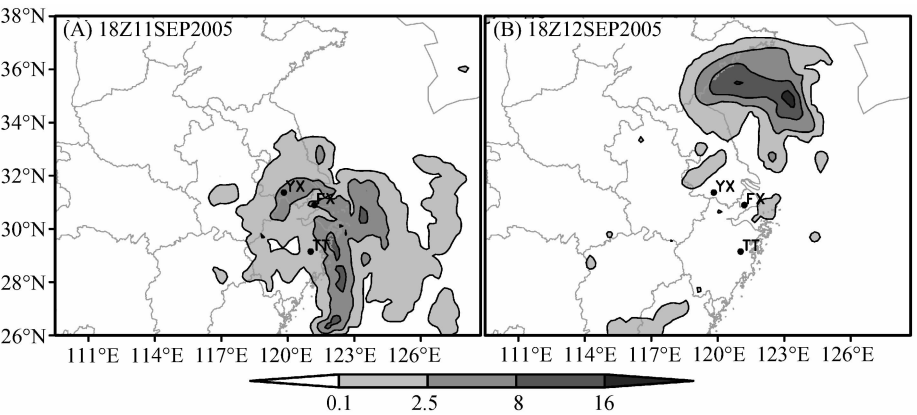
图 5 模拟褐飞虱起飞时刻(18:00)的降雨量 (Hu et al. , 2013) Fig.5 The simulated precipitation (mm) at 18:00 (Hu et al. , 2013) TT:天台 Tiantai;FX:奉贤 Fengxian;YX:宜兴 Yixing. A:2005 年 9 月 11 日 Sept. 11, 2005; B:2005 年 9 月 12 日 Sept. 12, 2005.
