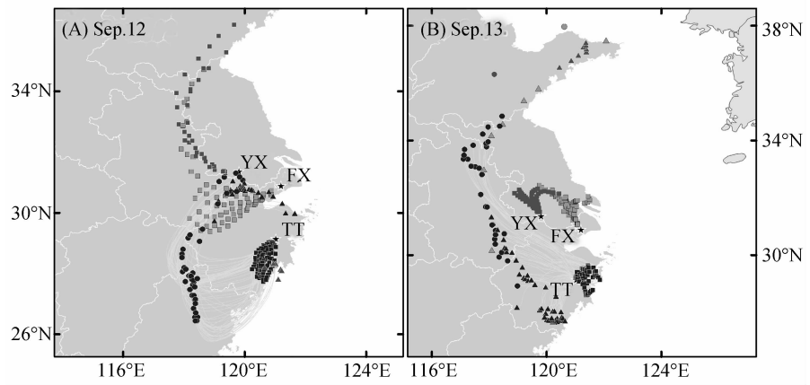
图 3 天台 (TT)、奉贤 (FX) 和宜兴 (YX) 褐飞虱 2005 年 9 月 12 (A)、13 日 (B) 的回推轨迹终点 (Hu et al. , 2013) Fig. 3 Endpoints of backward trajectories of Nilaparvate lugens starting from Tiantai (TT), Fengxian (FX) and Yixing (YX) during Sept. 12 (A) and 13 (B)
