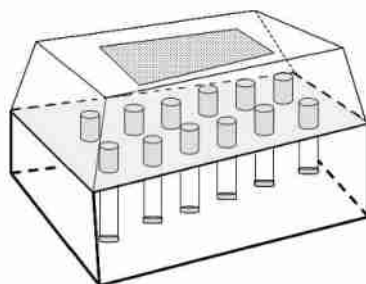
图 3 分隔式养虫笼整体透视图
