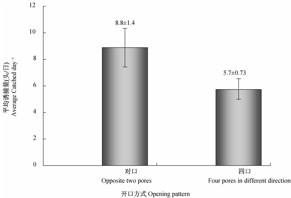
图 3 陷阱式诱捕器两种开口方式的诱捕效果比较
