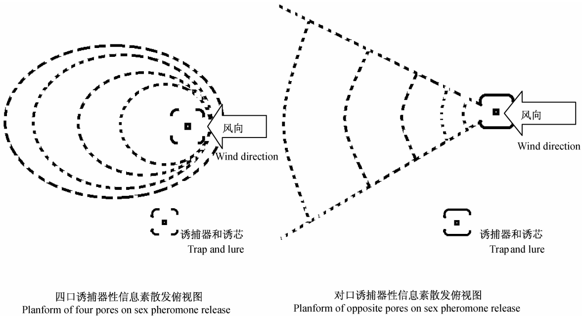
图 6 在风作用下不同开口方式的陷阱诱捕器的性信息素扩散 Fig. 6 The sex pheromone diffusion with different opening traps under the action of wind force
