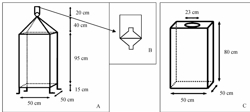
图 1 笼罩 (A)、采集瓶 (B)、吸虫罩 (C) 示意图
