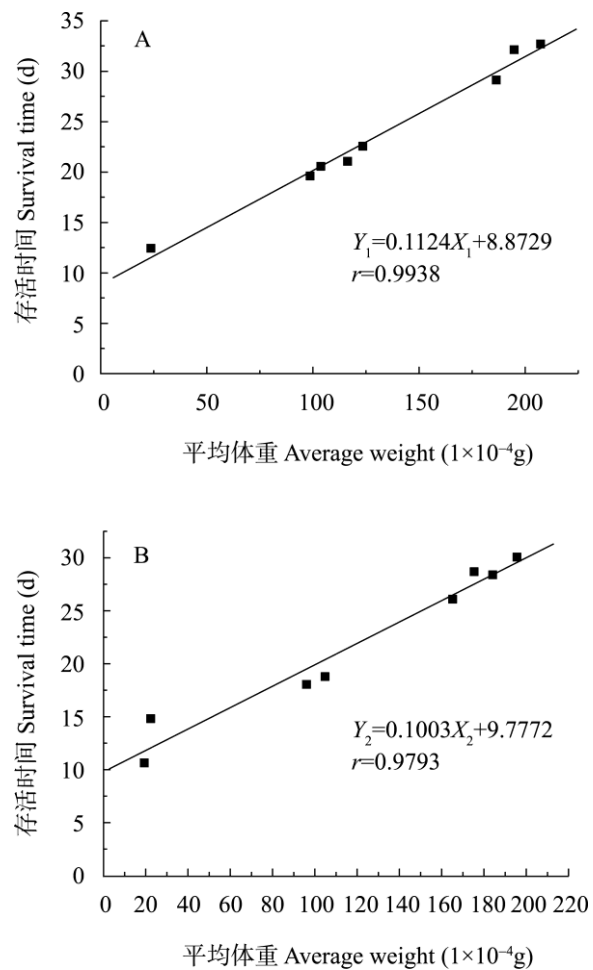
图 1 华丽肖蛸 (A) 和锥腹肖蛸 (B) 存活天数对体重的散点图及拟合回归线
