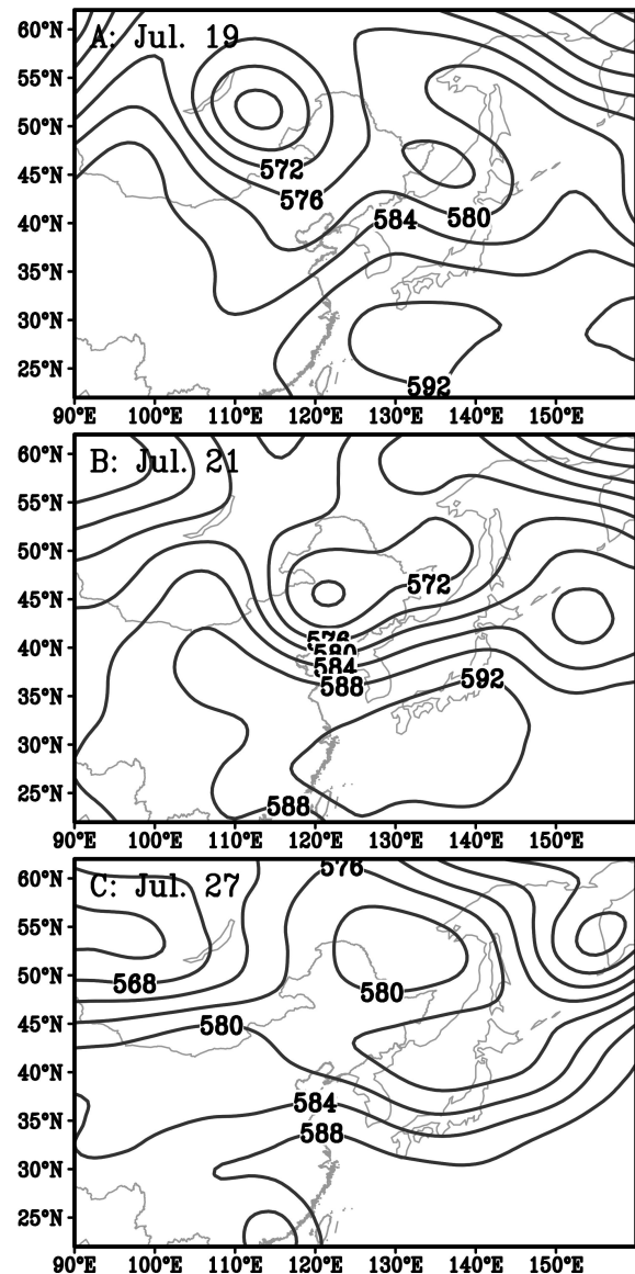
图4 1980年7月19、21、27日20:00我国东部地区500 hPa高度场
