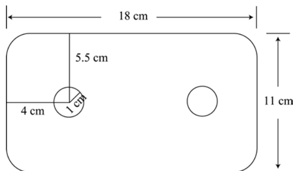
图 1 试验容器示意图
