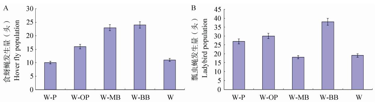
图 13 不同处理模式下两种天敌昆虫发生量 Fig. 13 Two natural enemies' population in the wheat field under different intercropping system (mean±SE) A: 食蚜蝇 Hoverfly B: 瓢虫 Ladybird; W-P: 小麦与大蒜间作 Wheat-garlic; W-OP: 小麦与油菜间作 Wheat -oil rape; W-MB: 小麦与绿豆间作 Wheat-mung bean; W-BB: 小麦与蚕豆间作 Wheat-broad bean; W: 小麦单作 Wheat monoculture.
