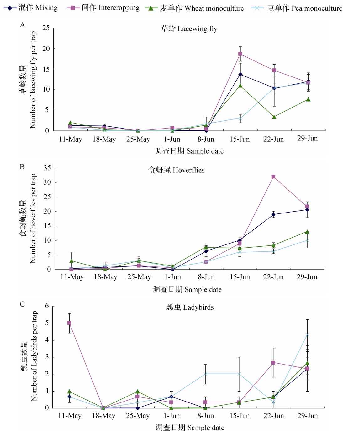
图 8 不同处理对天敌昆虫种群动态变化的影响
