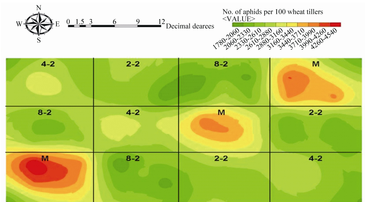
图 6 麦长管蚜发生高峰期的种群田间分布 GIS 图像 Fig. 6 GIS image of Sitobion avenae densities estimate during peak period
