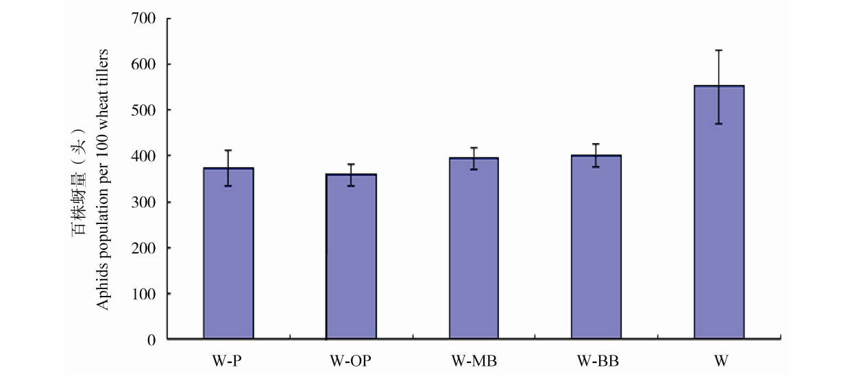
图 12 不同处理模式下麦蚜的平均百株蚜量 (mean±SE) Fig. 12 The average aphids population of per 100 wheat tillers under the different intercropping system (mean±SE) W-P: 小麦与大蒜间作 Wheat-garlic; W-OP: 小麦与油菜间作 Wheat-oil rape; W-MB: 小麦与绿豆间作 Wheat-mung bean; W-BB: 小麦与蚕豆间作 Wheat-broad bean; W: 小麦单作 Wheat monoculture.
