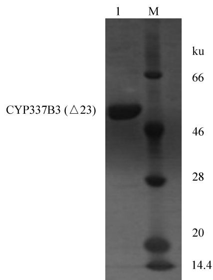
图 4 CYP337B3 ( \Delta 23 ) 蛋白纯化结果
