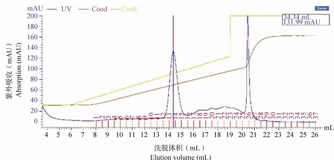
图 5 CYP337B3 ( \Delta 23 ) 蛋白 RESOURCE™ Q 离子交换层析图
