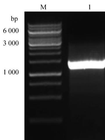
图 2 CYP337B3 ( \Delta 23 ) 基因 PCR 扩增结果
