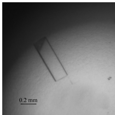
图 7 CYP337B3 ( \Delta 23 ) 蛋白晶体 Fig. 7 Typical crystals of CYP337B3 ( \Delta 23 )
