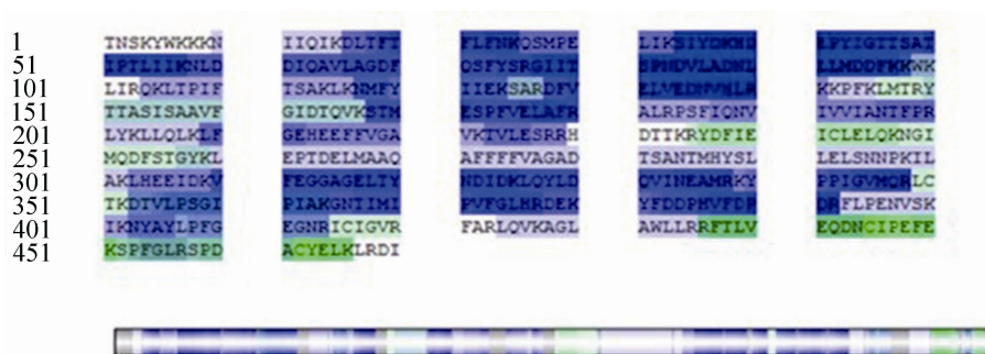
图 6 CYP337B3 ( \Delta 23 ) 蛋白质谱分析结果
