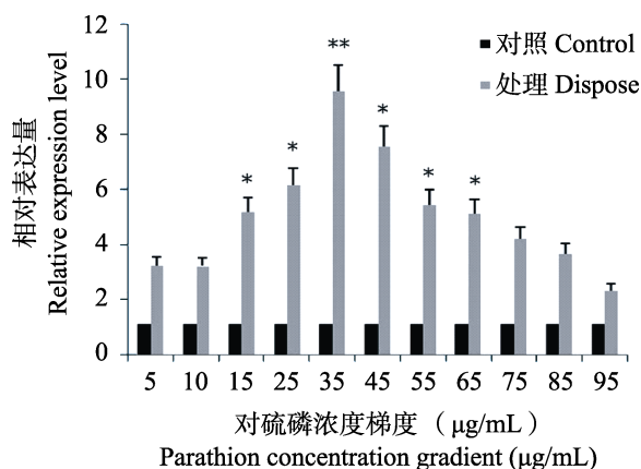
图4 不同浓度对硫磷处理细胞后 Cyp6a8 的表达量 Fig. 4 Different concentrations of parathion cells after the expression of Cyp6a8 expression
