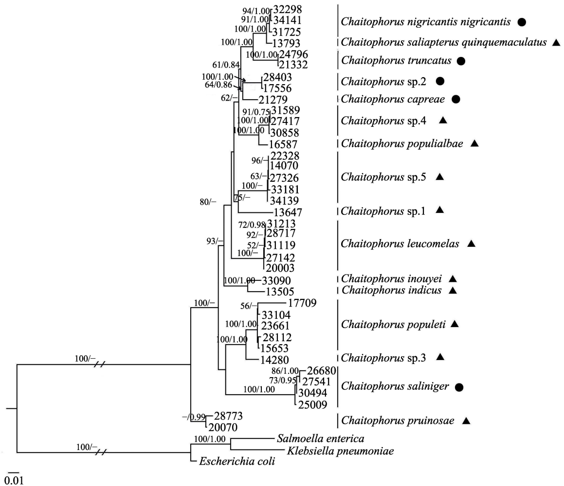
图 2 基于 atpD/gnd/trpB/16S rDNA 联合基因数据集构建的 Buchnera 最大似然树
