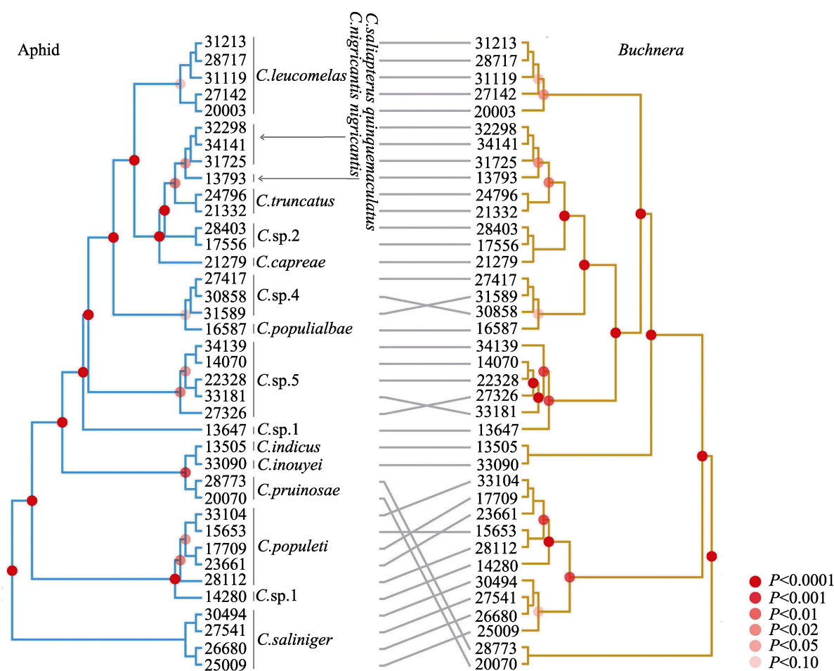
图 3 TreeMap 蚜虫- Buchnera 系统发育树对比图
