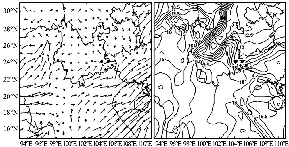
图 8 2010 年 5 月 29 日 800 hPa 高度上水平风场 (左) 和温度场 (右)
