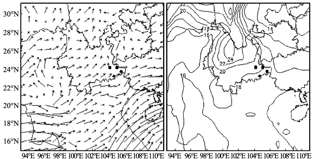
图 9 2010 年 5 月 30 日 800 hPa 高度上水平风场 (左边) 和温度场 (右边)
