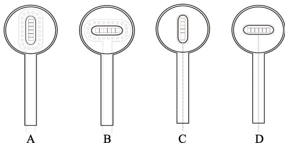
图7 不同捞片环将连续切片放置于位于放样孔内的狭缝载网上使用状态示意图
