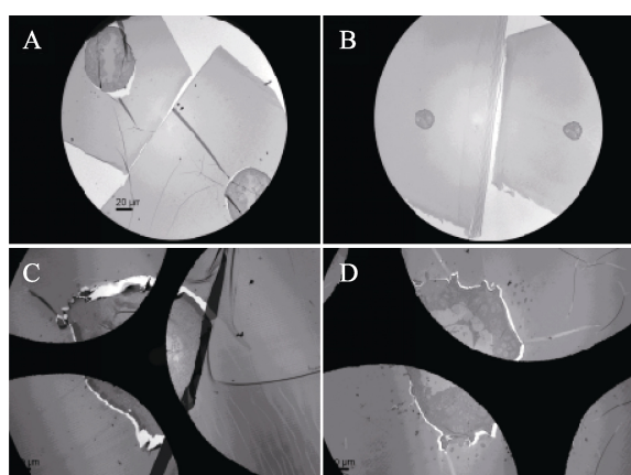
图 8 组合器具捞片与传统粘取式捞片结果对比
