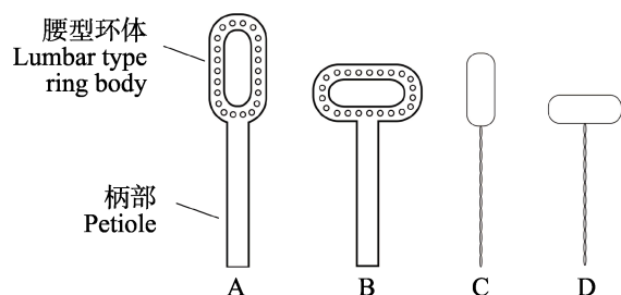
图6 捞片环结构示意图
