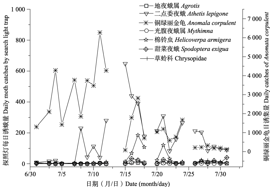
图 1 2 代二点委夜蛾发生期间探照灯诱集的主要昆虫群落数量(原阳, 2016)
