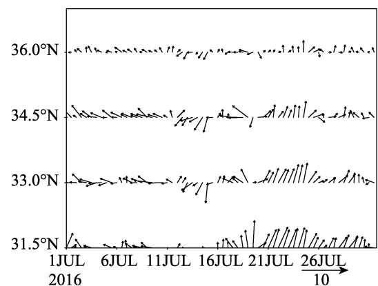
图 6 2016 年 7 月原阳监测点所在区域 950 hPa 高度沿 113.7°E 风场的时间-纬度剖面
