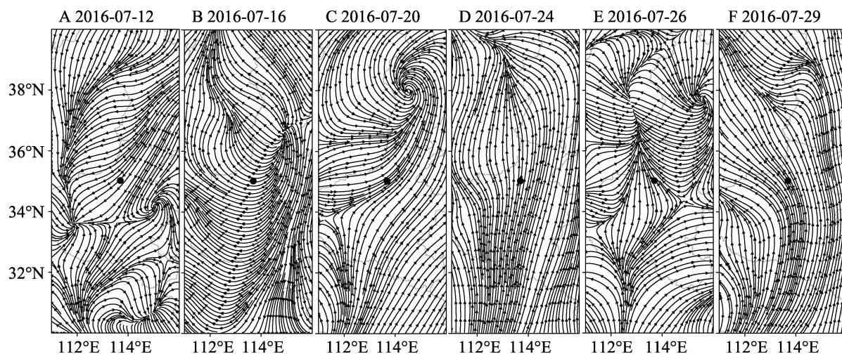
图7 2016年7月原阳监测点(黑点所示)所在区域上空950 hPa高度20:00流场分布 Fig. 7 Streamlines at 20:00 and 950 hPa in VLR site (the dot, YuanYang) in July 2016
