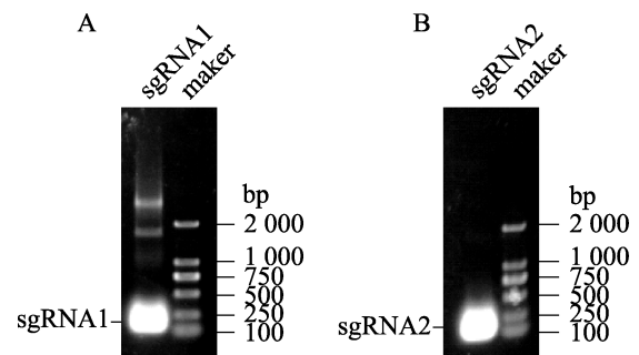
图 3 sgRNA1 (A) 和 sgRNA2 (B) 同源片段的 PCR 扩增
