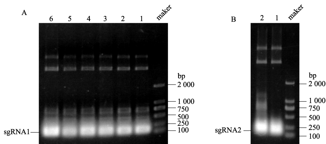
图 5 PCR 扩增验证 sgRNA 表达载体的构建
