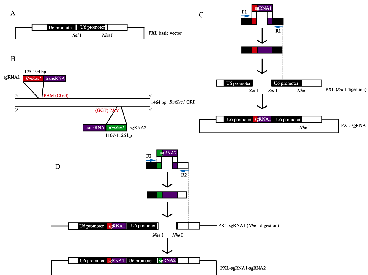
图 1 表达二元 sgRNA 的 CRISPR 载体的构建示意图
