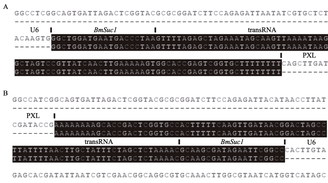
图 4 TA 克隆测序验证 sgRNA 同源片段的序列
