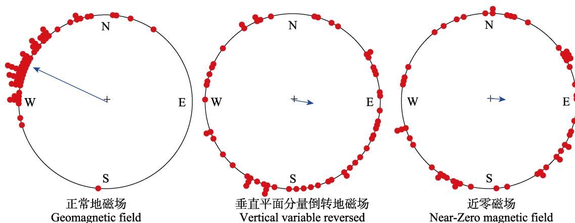
图3 正常地磁场条件下饲养的粘虫在不同磁场中的共同定向行为
