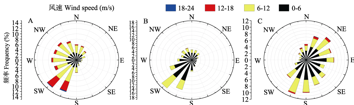
图 3 9 月 925 hPa 风玫瑰图 (1957-2001)
