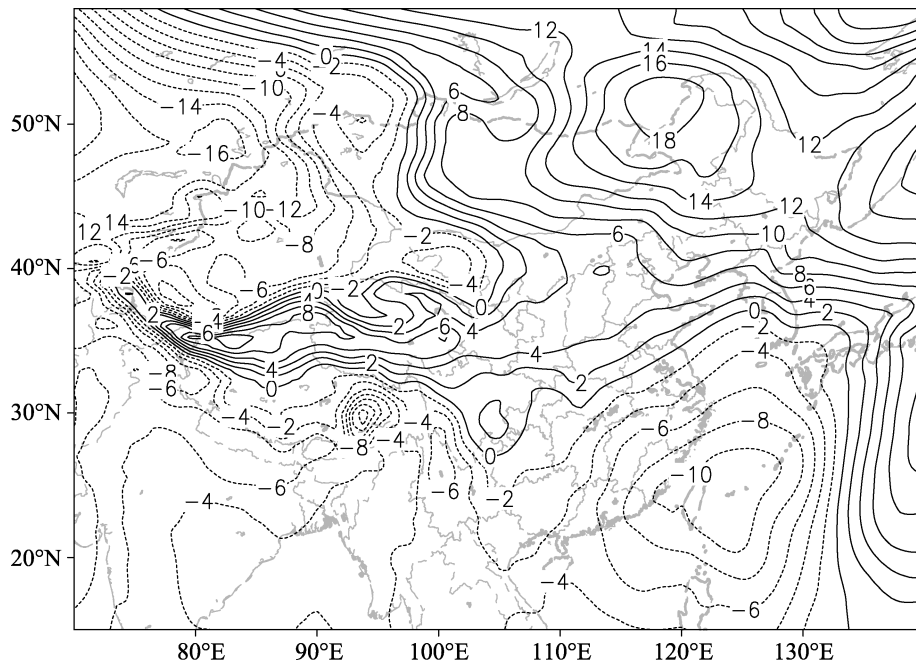
图 5 重发生年与轻发生年的上年 9 月 925 hPa 高度场差值图
