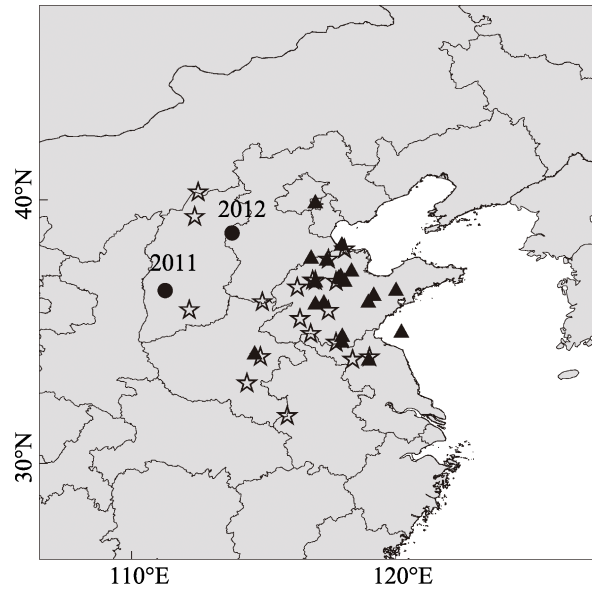
图 4 1960-1998 年各年 9 月 925 hPa 冷高压中心的位置
