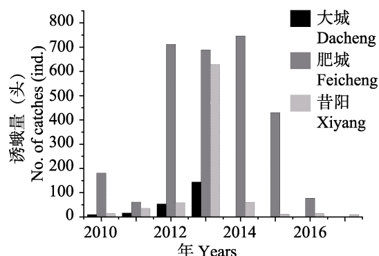
图 1 河北大城、山东肥城和山西昔阳 1 代粘虫总诱蛾量 (2010-2017)
