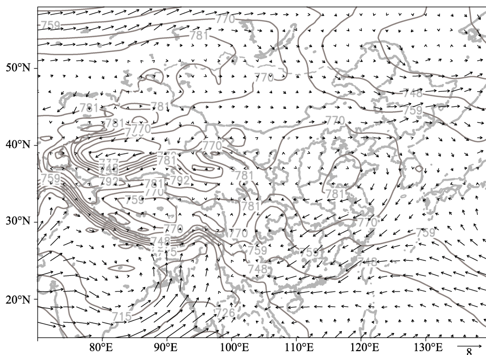
图 2 9 月 925 hPa 平均风场和高度场 (1957-2001)
