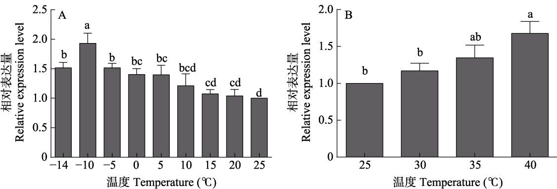
图 6 GdTPP 在沙葱萤叶甲 2 龄幼虫不同温度胁迫下的相对表达量
