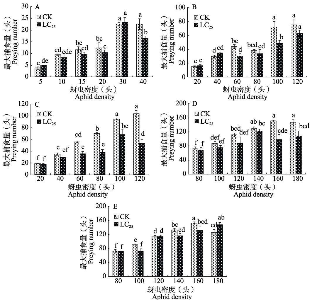
图 2 不同虫态的异色瓢虫对蚜虫的的捕食量
