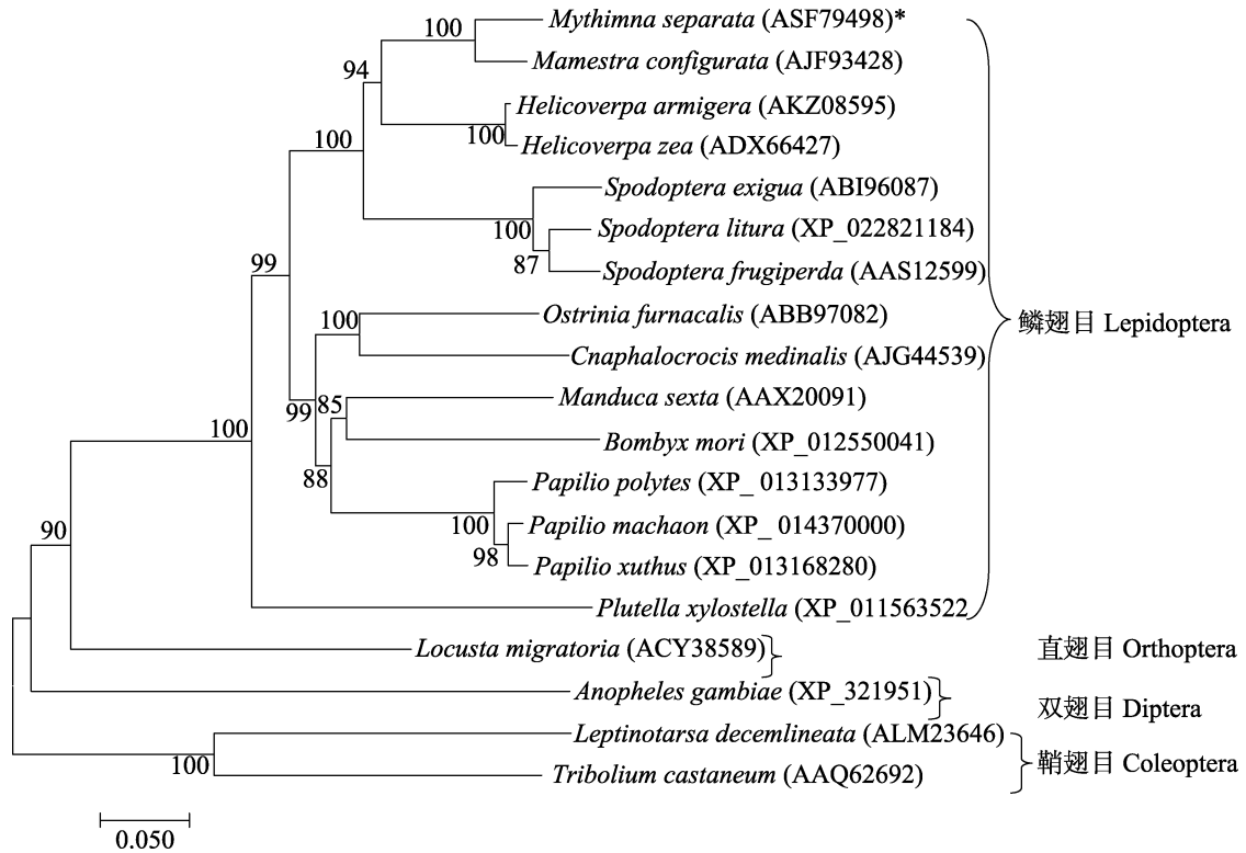
图 2 利用邻近法构建的昆虫 CHSB 氨基酸序列系统进化树
