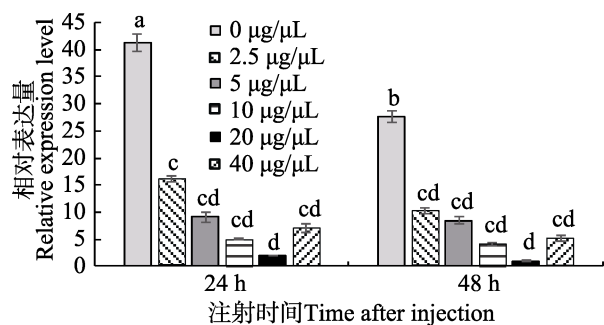
图6 有效霉素诱导下 MsCHSB 相对表达量
