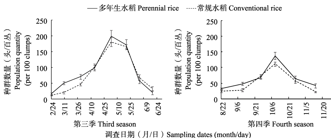
图 5 二季稻区多年生水稻及常规水稻田间主要害虫种群动态
