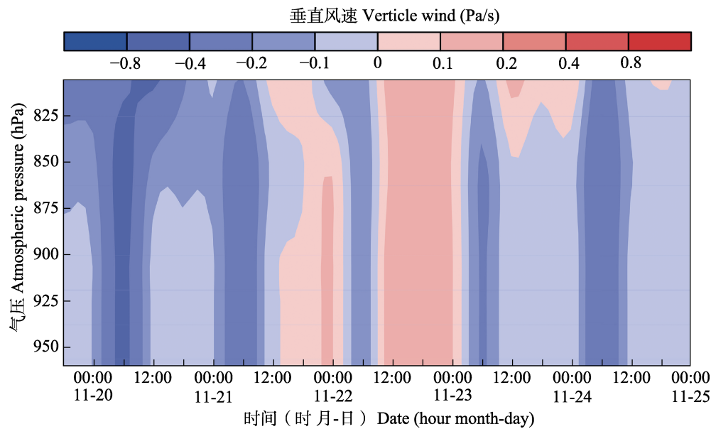
图 4 2018 年 11 月 19-25 日江城地区 800-950 hPa 垂直风场的时间-高度剖面图
