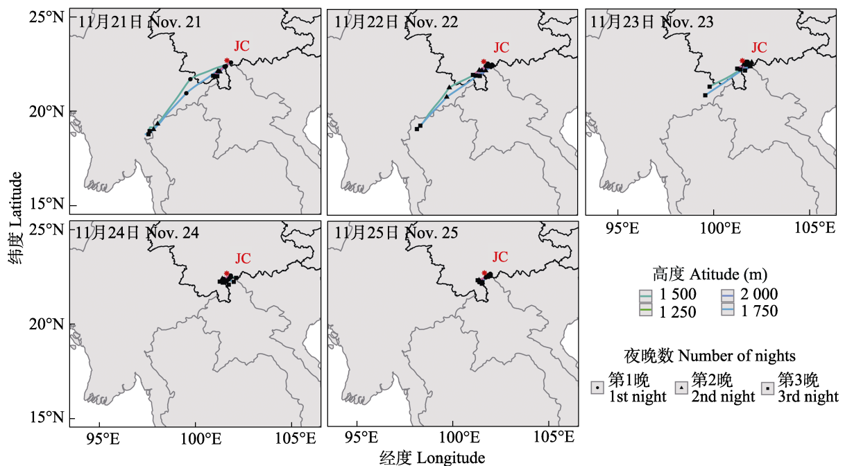
图 5 2018 年 11 月 21-25 日云南省江城县草地贪夜蛾回推轨迹分析
