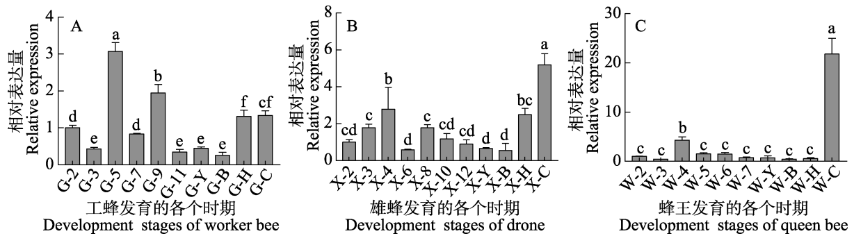
图 7 amPFK 基因不同品级不同发育时期的相对表达
