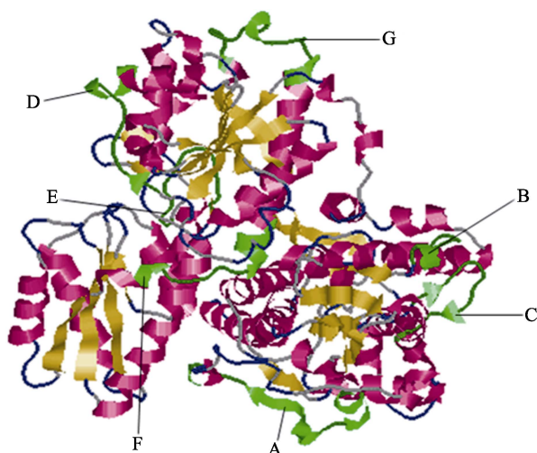
图4 意大利蜜蜂 amPFK 蛋白三级结构 (绿色部分为 B 细胞抗原表位)
