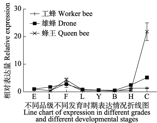
图 8 amPFK 基因在意大利蜜蜂不同品级不同发育时期表达情况折线图
