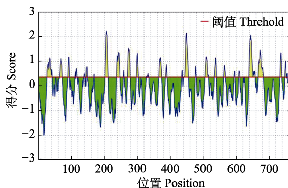
图5 amPFK 蛋白 B 细胞抗原表位分析
