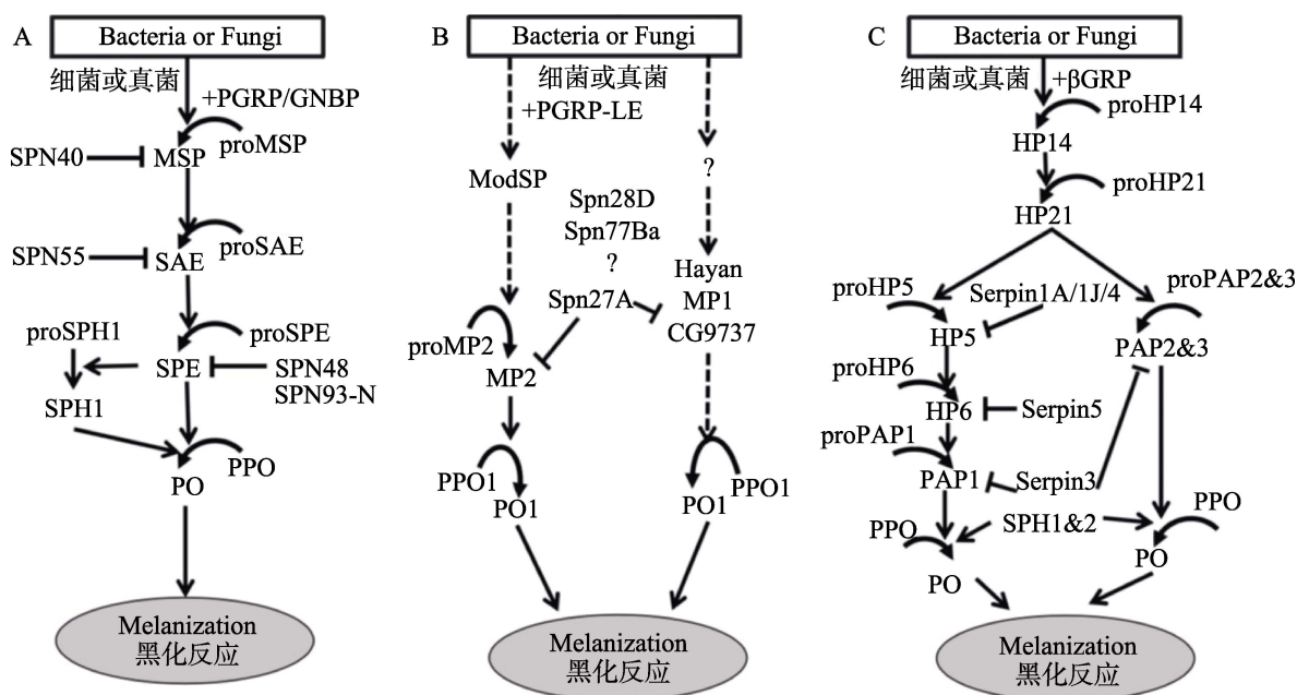
图3 昆虫中丝氨酸蛋白酶抑制剂对 PPO 激活通路的调控模式 (An et al. , 2013; Wang et al. , 2020)
