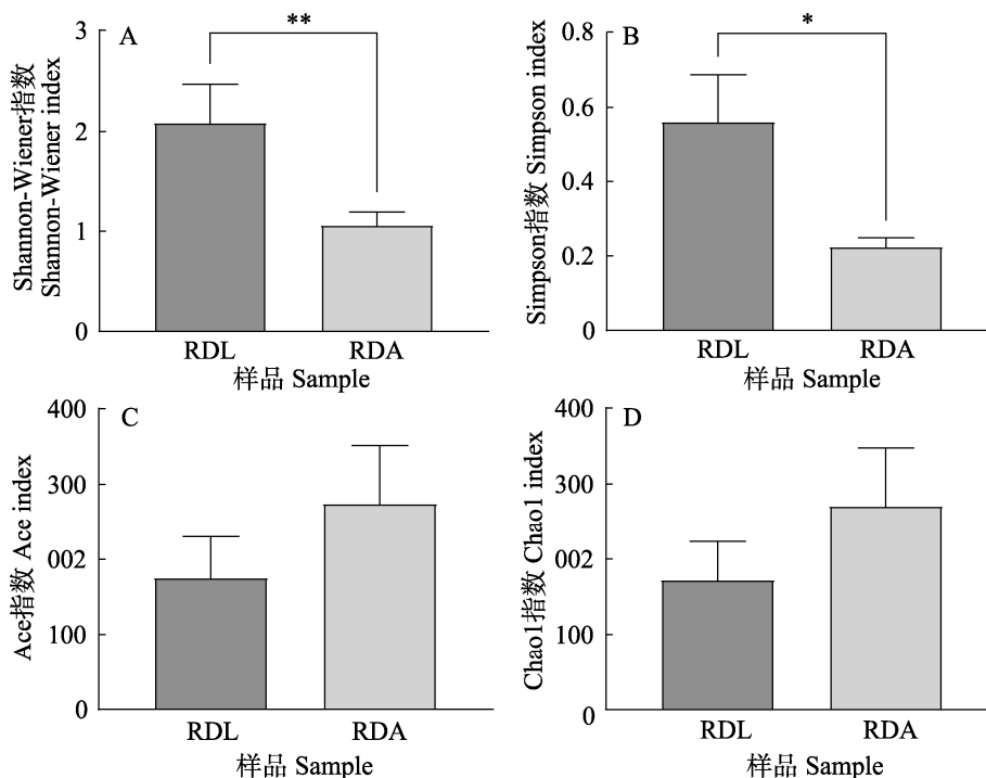
图 2 谷蠹幼虫和成虫体内细菌 \alpha 多样性指数差异分析
