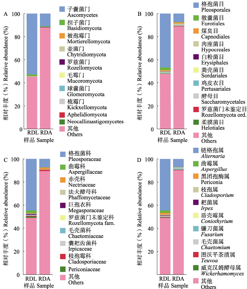
图 5 谷蠹幼虫和成虫体内真菌在门 (A)、目 (B)、科 (C) 和属 (D) 水平的相对丰度 Fig. 5 Relative abundance of the fungus at the phylum (A), order (B), family (C) and genus (D) levels in larvae and adults of Rhyzopertha dominica
