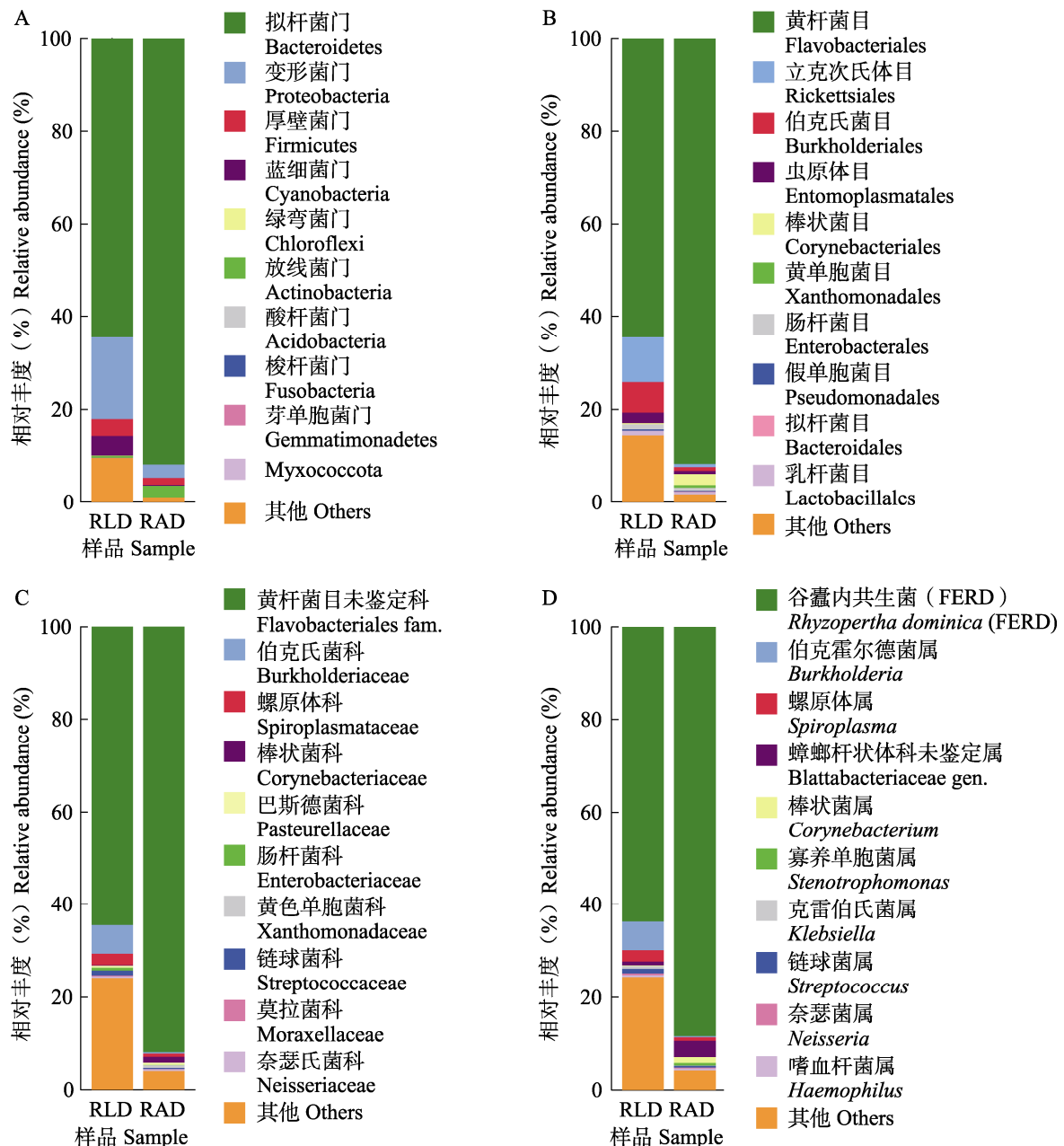
图 1 谷蠹幼虫和成虫体内细菌在门 (A)、目 (B)、科 (C) 和属 (D) 水平的相对丰度
