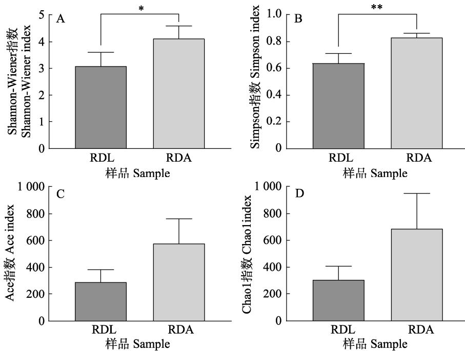
图 6 谷蠹幼虫和成虫体内真菌 \alpha 多样性指数差异分析
