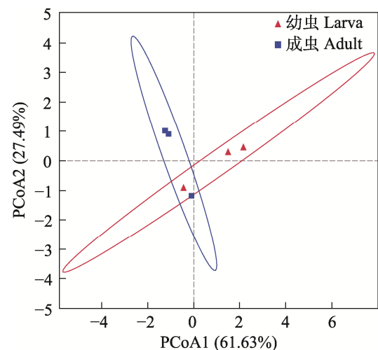
图 7 谷蠹幼虫和成虫体内真菌主坐标分析
