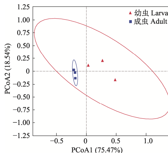
图 3 谷蠹幼虫和成虫体内细菌主坐标分析
