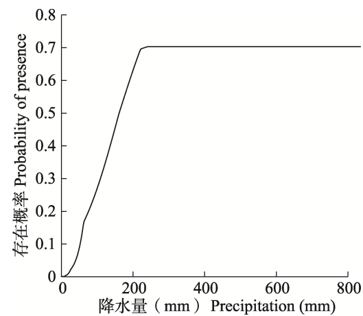
图 3 最冷季平均降水量 (bio19) Fig. 3 Mean precipitation of the coldest quarter
