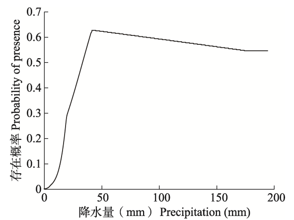
图 2 最干月份降水量 (bio14) Fig. 2 Precipitation of the driest month
