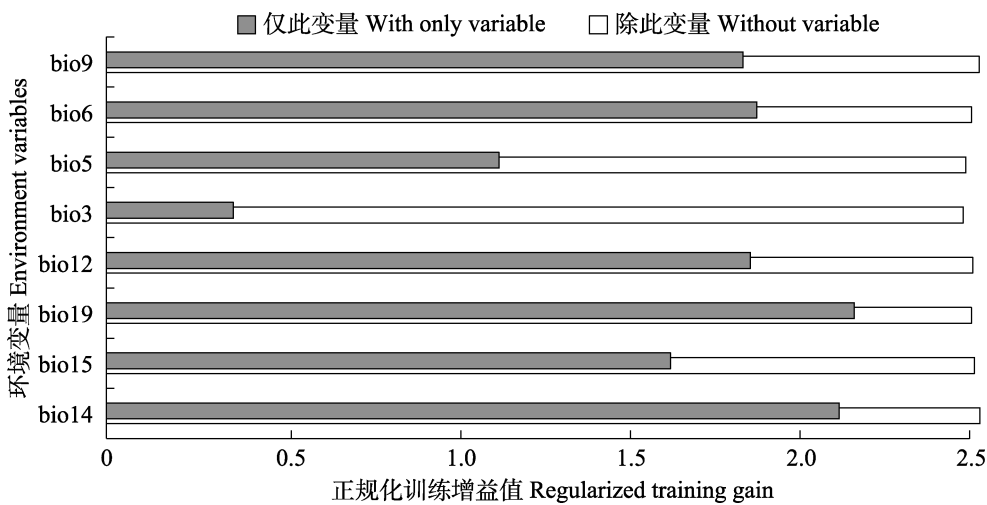
图 1 主导环境变量刀切法检验 Fig. 1 Jackknife test for evaluating the main environmental variables
