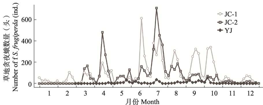
图 1 2020 年云南南部 3 个高空灯草地贪夜蛾每 5 日诱集虫量
