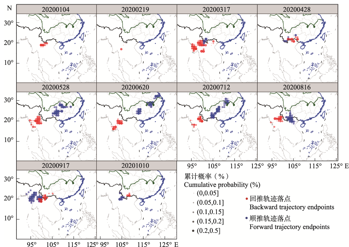
图 3 2020 年 1-10 月云南南部草地贪夜蛾顺推轨迹及回推轨迹落点分布
