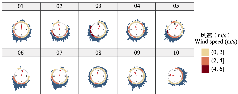
图 5 2020 年云南监测点 1-10 月 850 hPa 风向风速频次图
