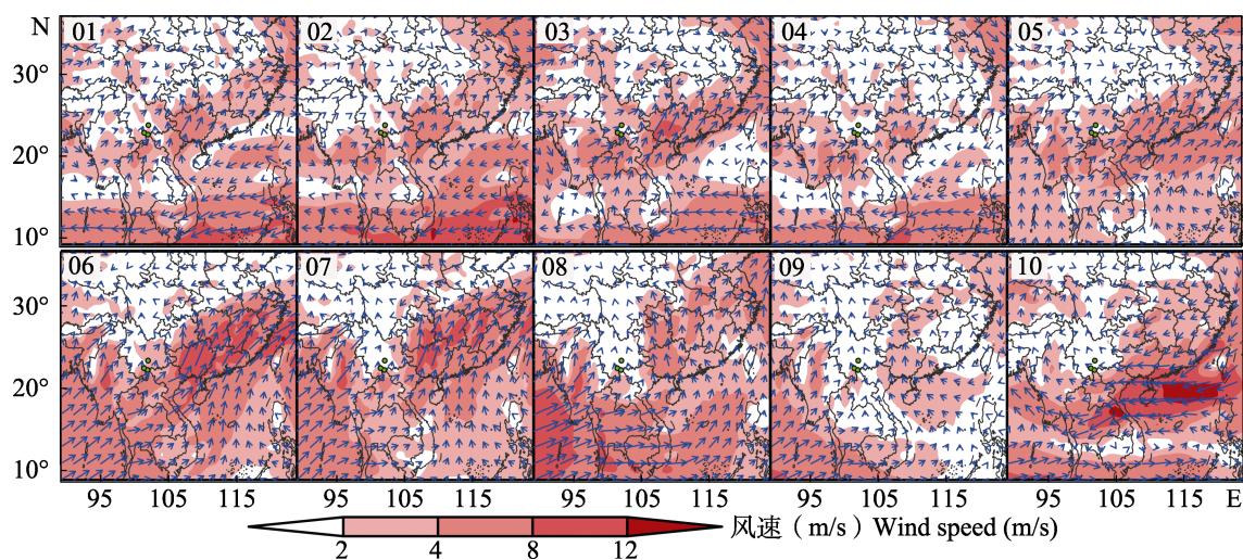
图 4 2020 年云南南部 1-10 月 850 hPa 平均风场
