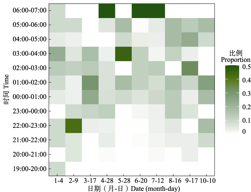
图 2 云南南部 3 个高空灯每月逐小时草地贪夜蛾灯诱比例
