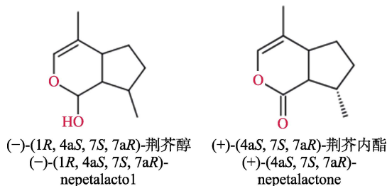
图 2 蚜虫性信息素两种主要成分分子结构示意图
