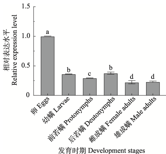
图4 FABP 基因在柑橘全爪螨生长发育不同阶段的相对表达水平
