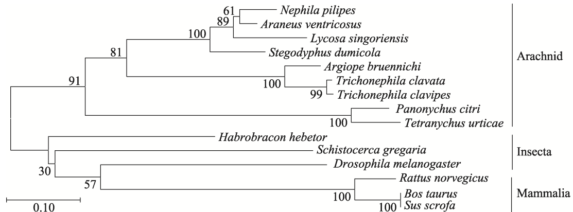
图3 以邻接法构建柑橘全爪螨 PcFABP 与其相关 FABPs 的系统发育树
