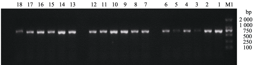
图 2 新鲜样本中 3 种方法提取的基因组 DNA 的 PCR 电泳结果 Fig. 2 PCR electrophoresis results of genomic DNA extracted by three methods in fresh samples
