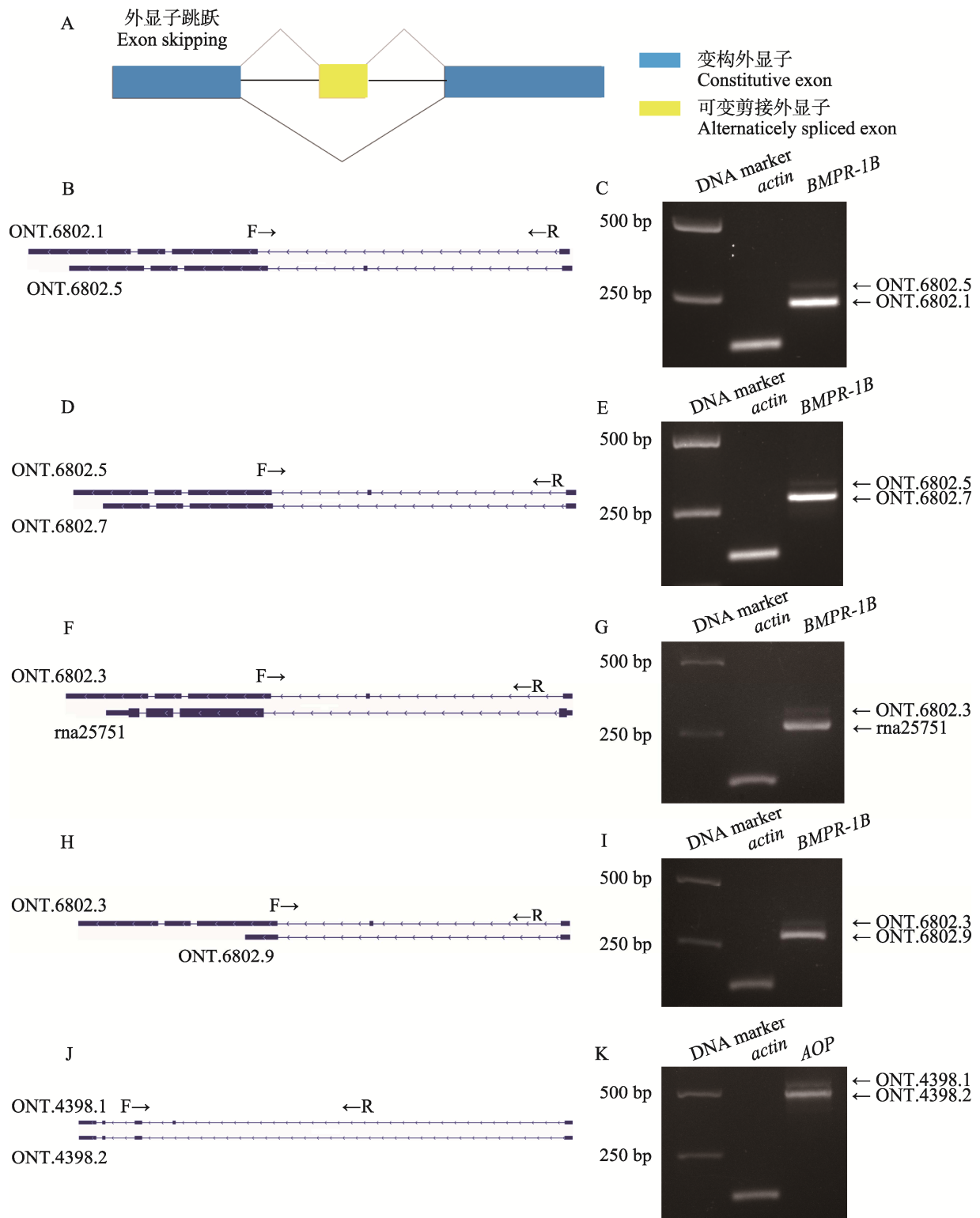
图 2 意大利蜜蜂 MAPK 信号通路相关的 2 个基因的 AS 事件验证
