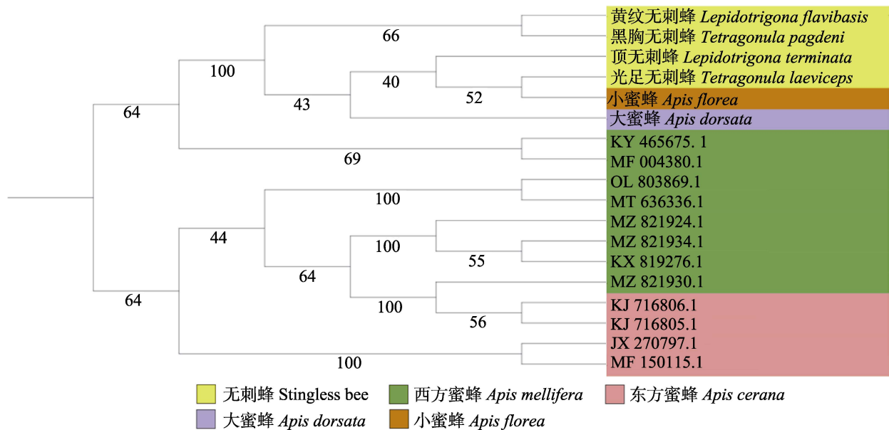
图 2 8 种寄主蜂种 SBV 毒株系统进化关系 Fig. 2 Evolutionary relationships of SBV taxa
