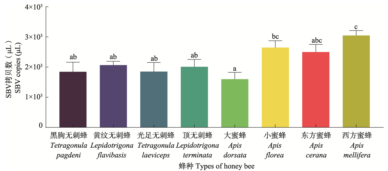
图 1 6 种野生蜂和 2 种饲养蜂种工蜂样本的 SBV 拷贝量差异性分析 Fig. 1 SBV copy quantity difference among six wild bee and two domestic bees
