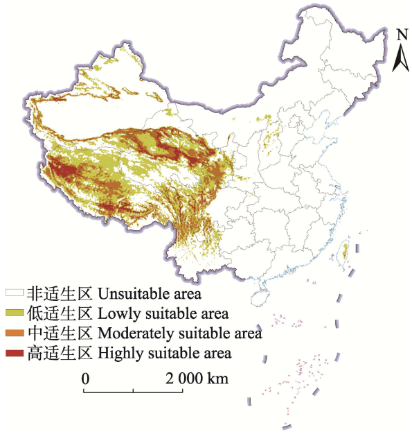
图 5 未来气候高强迫 SSP585 情景（2041-2060 SSP585）下苜蓿切叶蜂在中国的潜在地理分布 [审图号：京审字（2024）G 第 1860 号] Fig. 5 Potential geographical distribution in China of Megachile rotundata under future climatic conditions of high forcing scenarios (2041-2060 SSP585)
