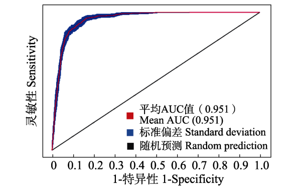
图 2 MaxEnt 模型对预测结果的 ROC 曲线及 AUC 值 Fig. 2 ROC curves and AUC values of predicted results of the MaxEnt model
