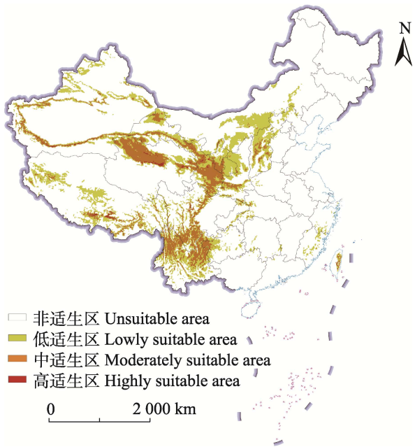
图 3 历史气候情景（1970-2000）下苜蓿切叶蜂在中国的潜在地理分布 [审图号：京审字（2024）G 第 1860 号] Fig. 3 Potential geographical distribution in China of Megachile rotundata under historical climatic scenarios (1970-2000)
