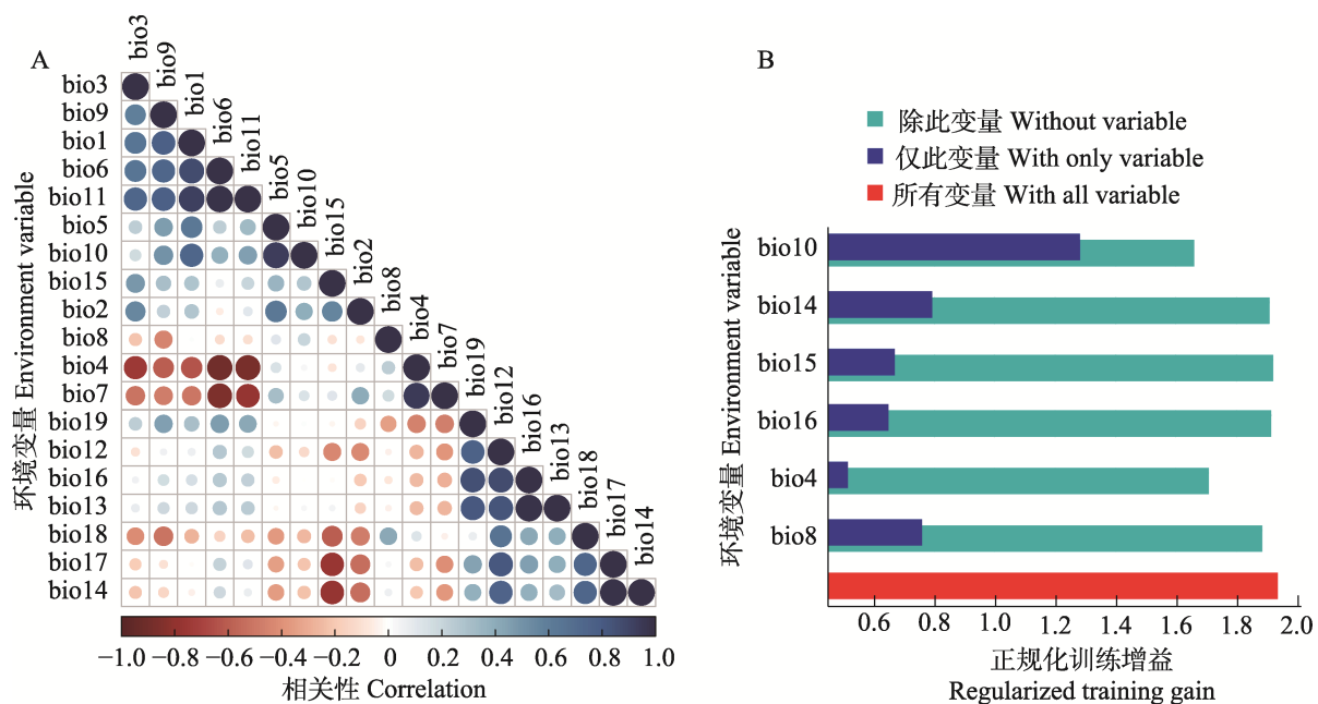
图 1 苜蓿切叶蜂环境变量筛选及贡献程度
