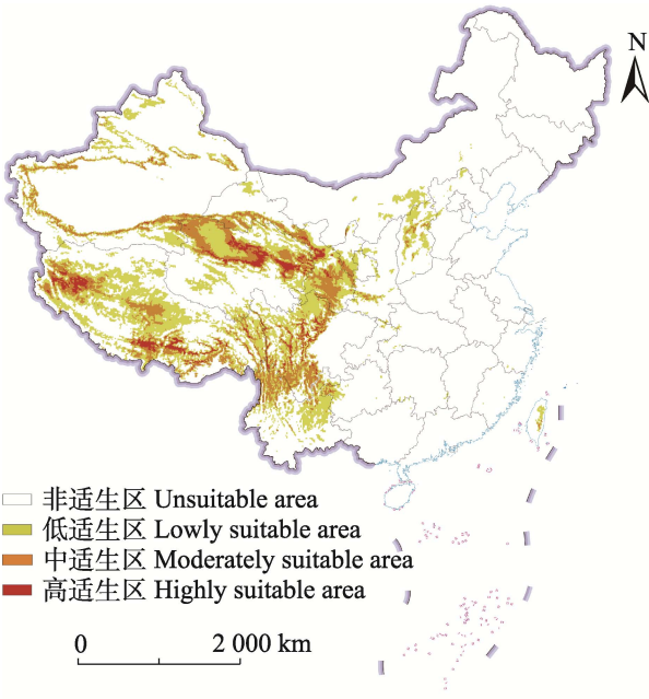
图 4 未来气候低强迫 SSP126 情景（2041-2060 SSP126）下苜蓿切叶蜂在中国的潜在地理分布 [审图号：京审字（2024）G 第 1860 号] Fig. 4 Potential geographical distribution in China of Megachile rotundata under future climatic conditions of low forcing scenarios (2041-2060 SSP126)
