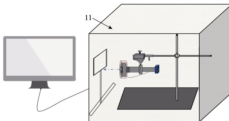
图 3 产卵行为观测装置连接顺序
