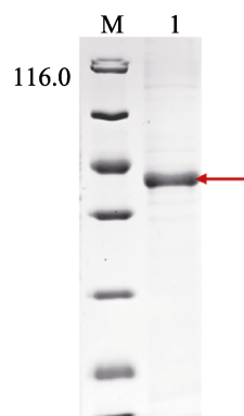
图 7 洗脱蛋白的 SDS-PAGE 电泳图 Fig. 7 SDS-PAGE Electrophoretogram of elution proteins
