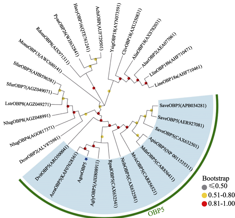
图4 基于枸杞棉蚜 AgosOBP5 氨基酸序列构建的昆虫 OBPs 进化树
